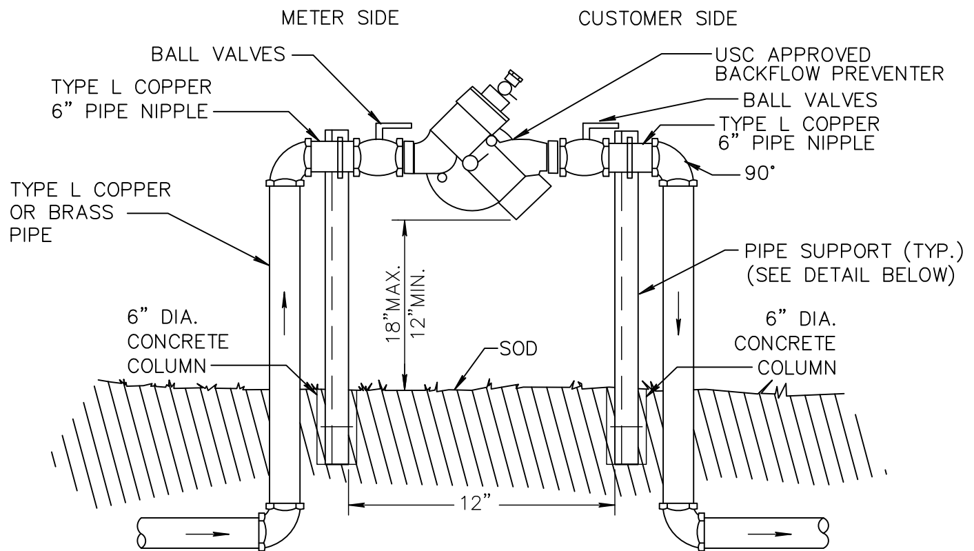
ELEVATION
