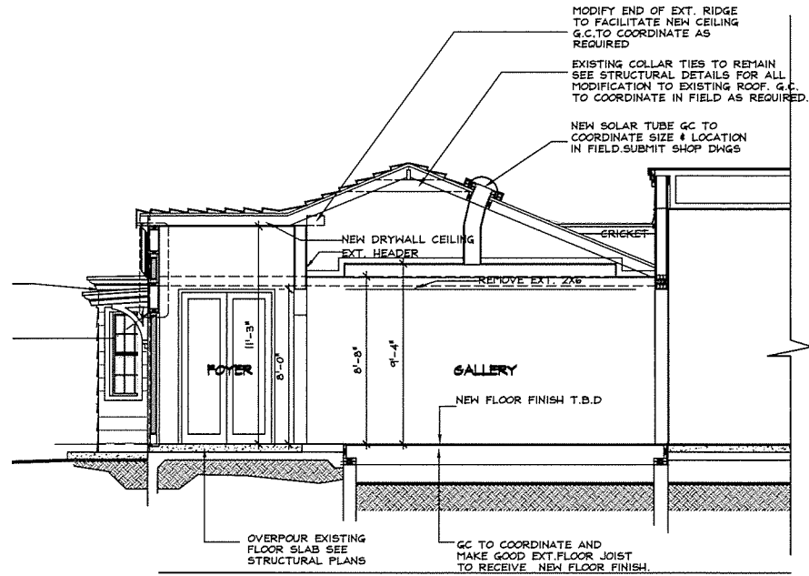
SECTION 'B'
