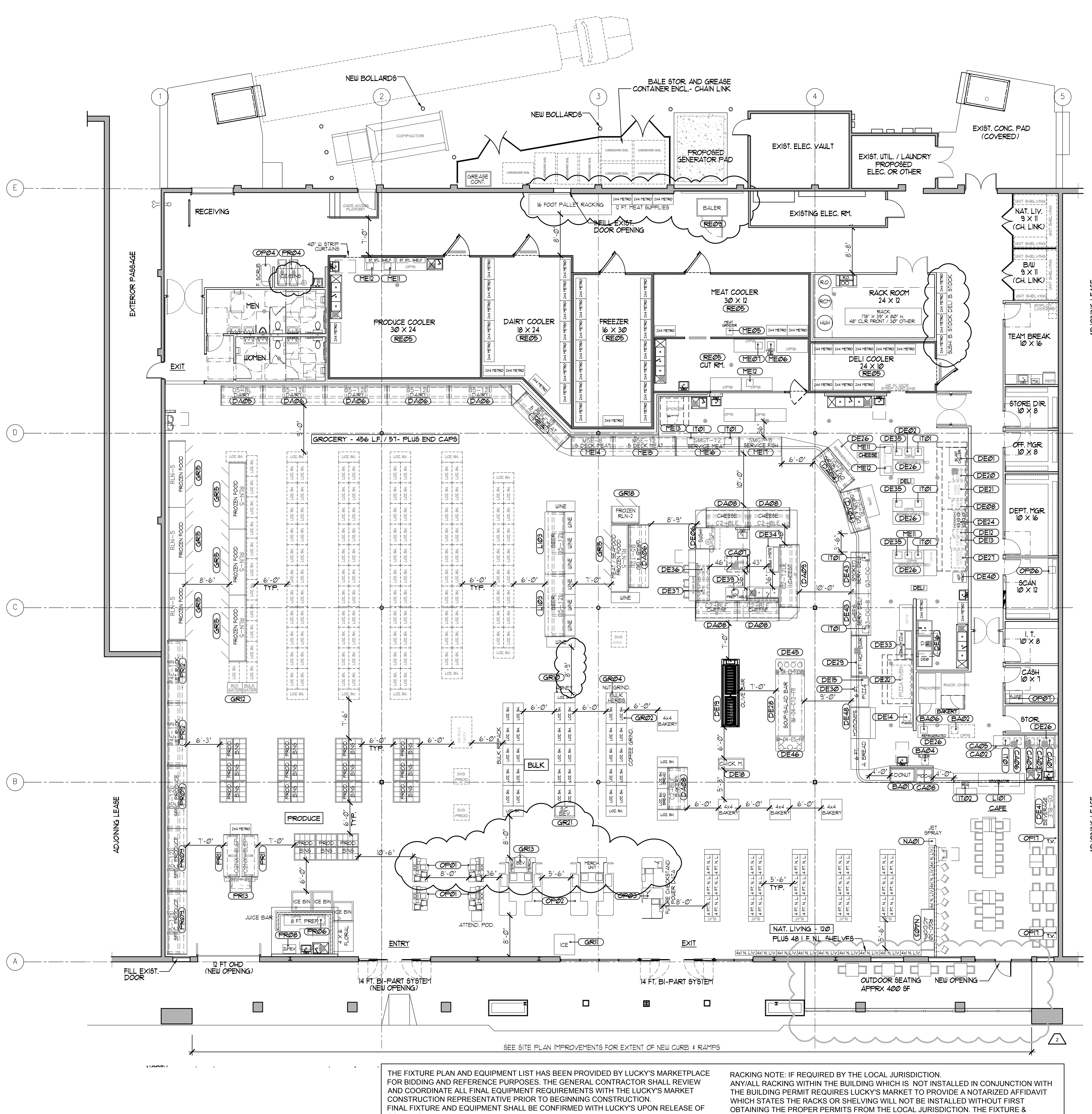
01 FIXTURE PLAN SCALE: 1/8" = 1'-0"
